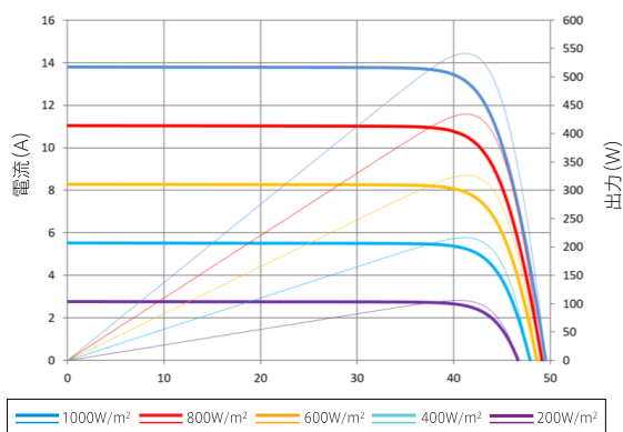
電流-電圧及び出力-電圧曲線 (STP540S-C72/Pmh+)
