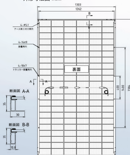
外形寸法図 単位:mm
